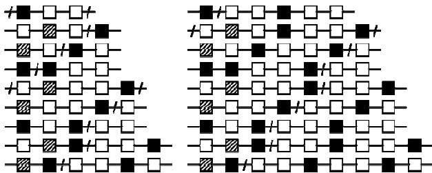
Fig. 3. Funcionamento da máquina exponencial inexata estudada. Os quadrados representam as funções adaptativas de cada transição. A aresta cortada indica um estado final.
